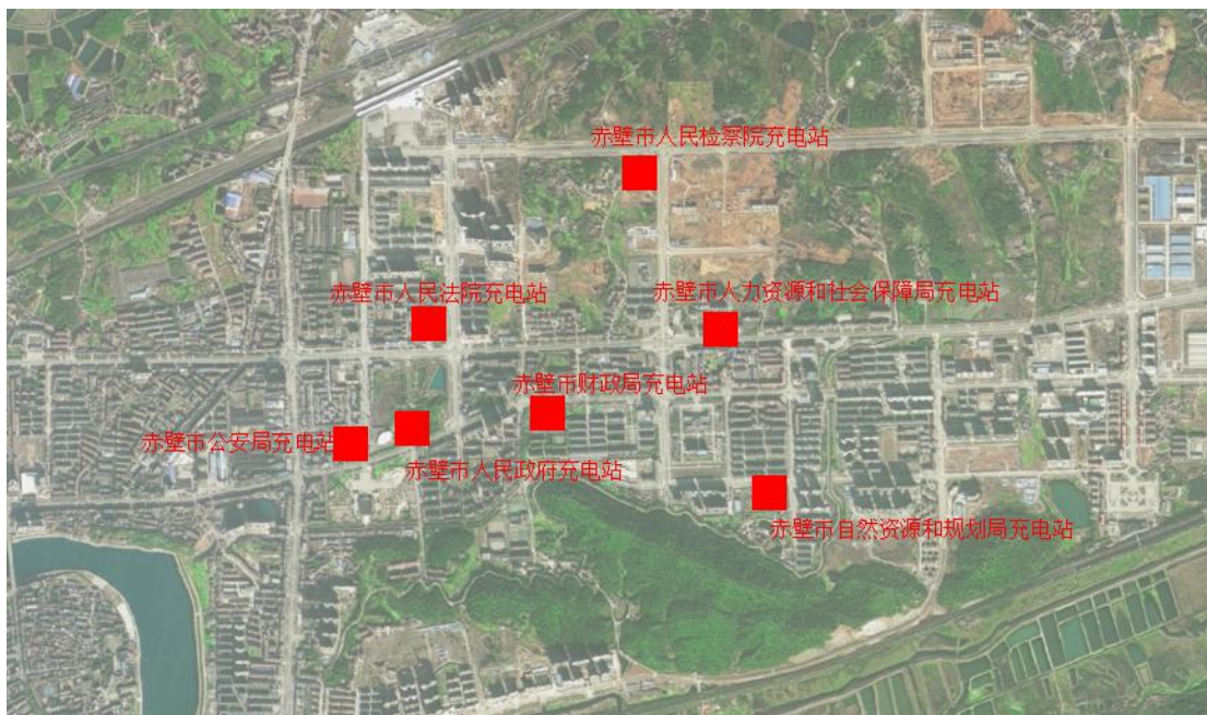
图 4- 54 赤壁市城区公务充电站布局规划图
