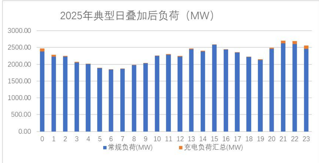
图 4- 125 咸宁市 2025 年典型日叠加负荷
