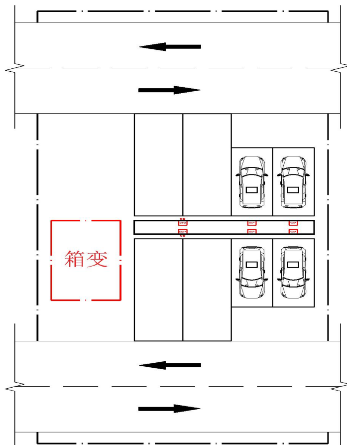
图 4 8 车位双排充电站布置图
