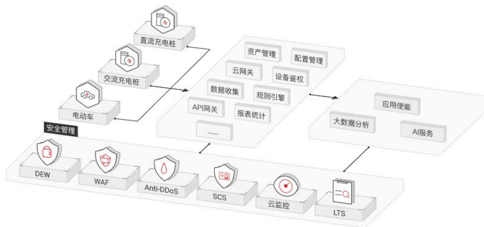
图 4- 126 咸宁市智慧运管云平台架构图
