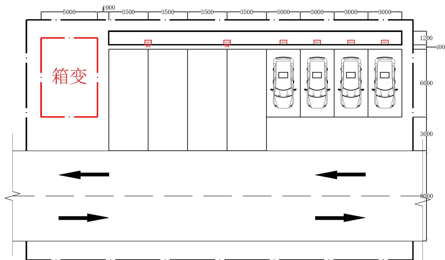
图 3 8 车位单排充电站布置图
