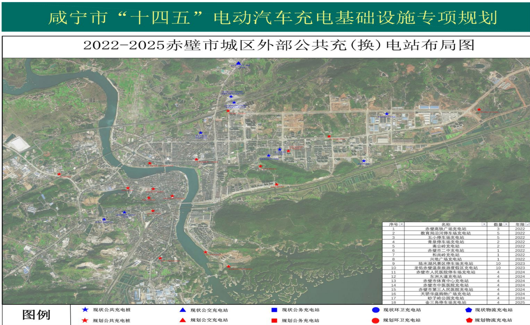
附图8 咸宁市各县市外部公共充（换）电站近期建设规划图
