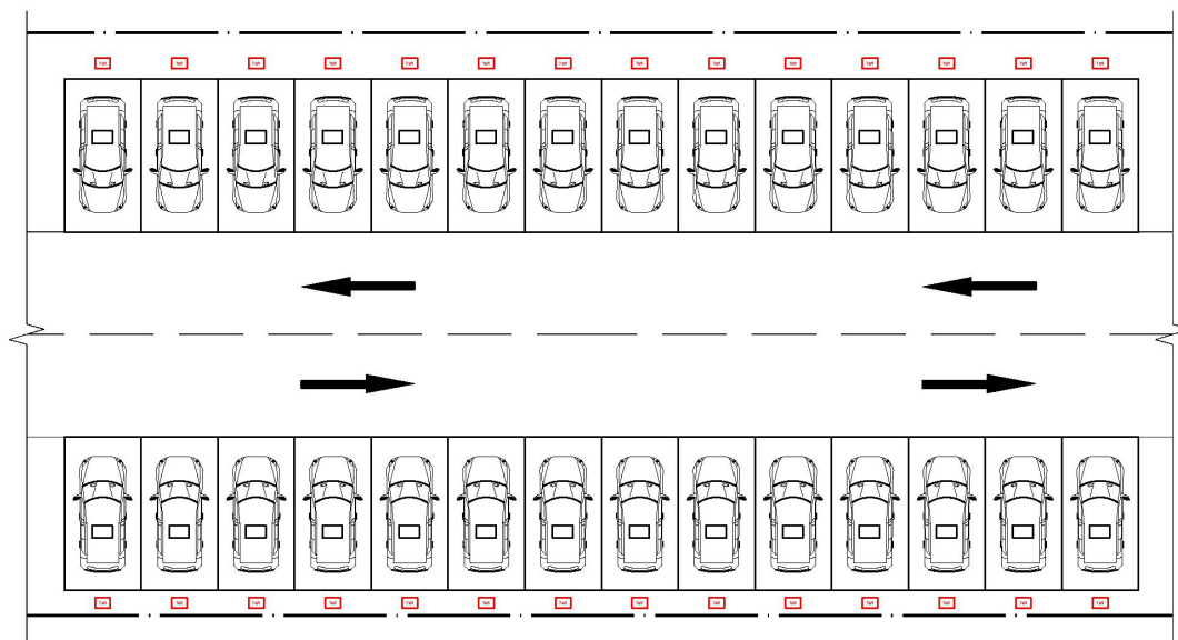
图 9 居民小区地下充电站布置图
