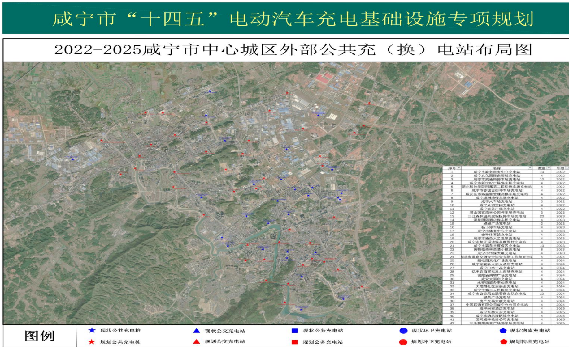
附图7 咸宁市中心城区外部公共充（换）电站近期建设规划图
