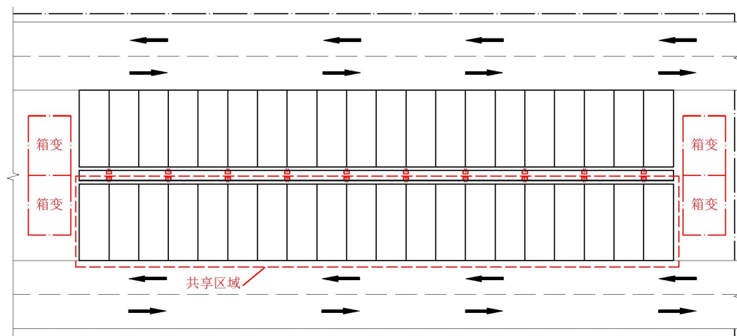
图 5 城市公交车充电站布置图
