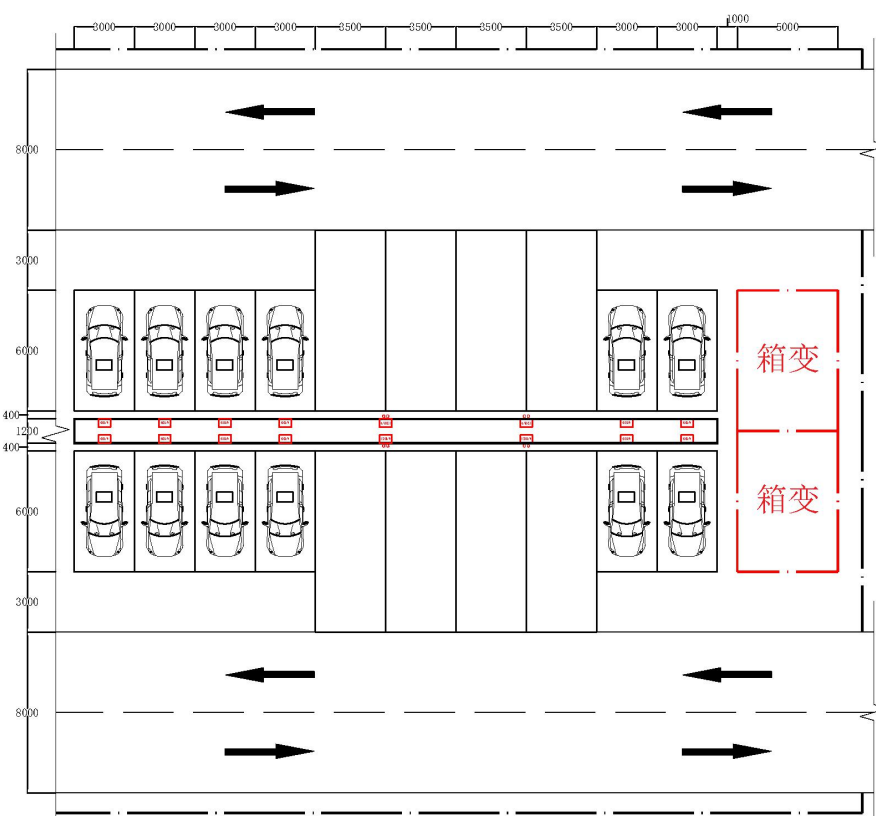
图 6 物流园充电站双排布置图
