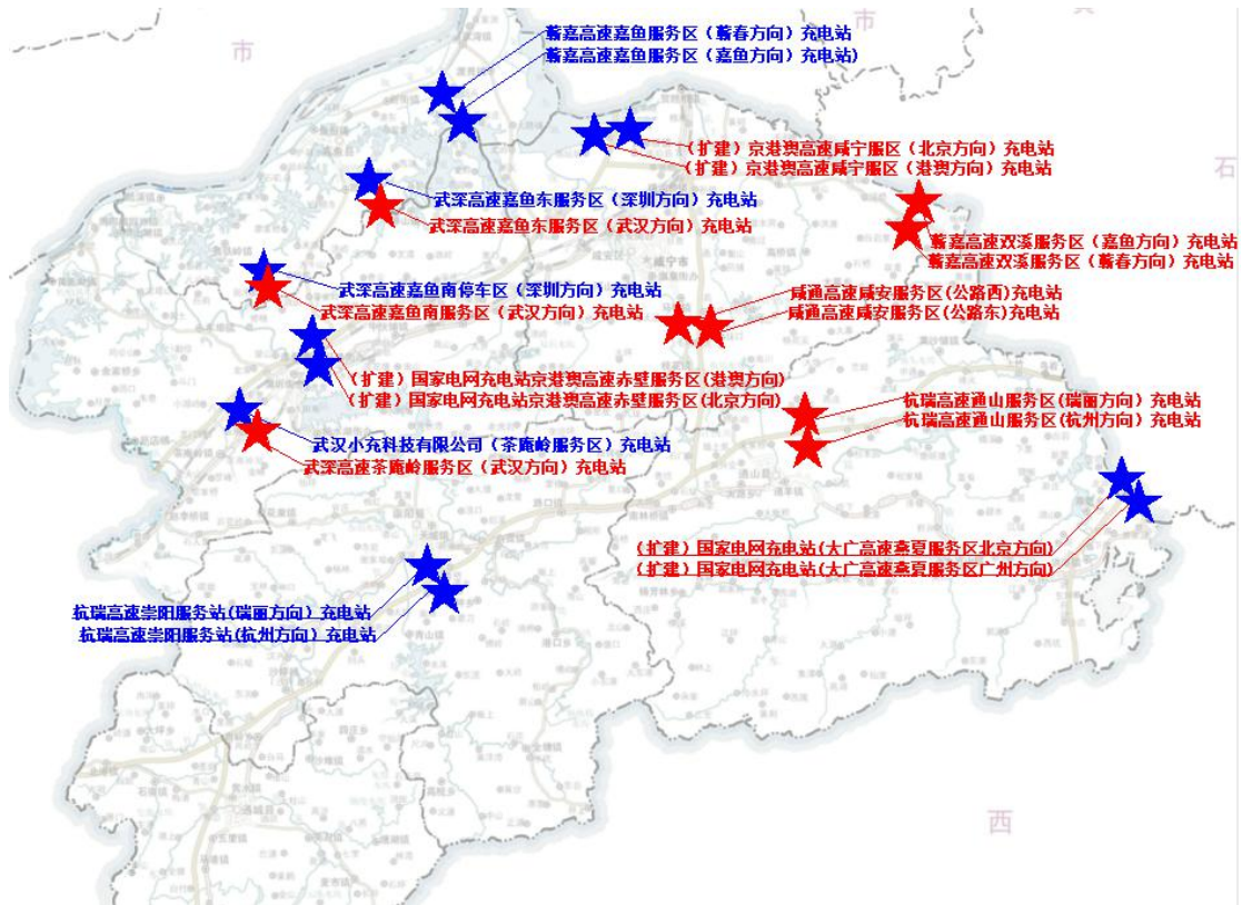
图 4- 2 咸宁市高速充（换）电站布局规划图
