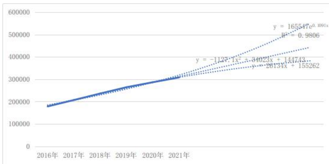
图3-11 回归曲线图
