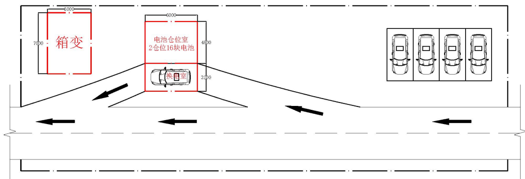
图 2 换电站布置图
