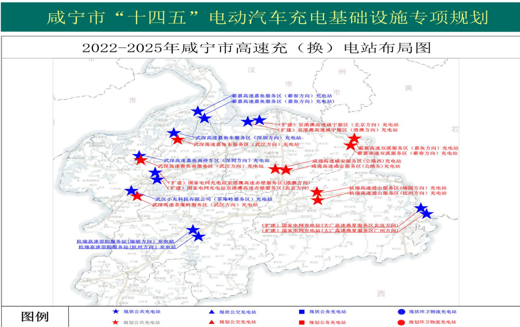
附图2 2022-2025年咸宁市高速充（换）电站布局图
