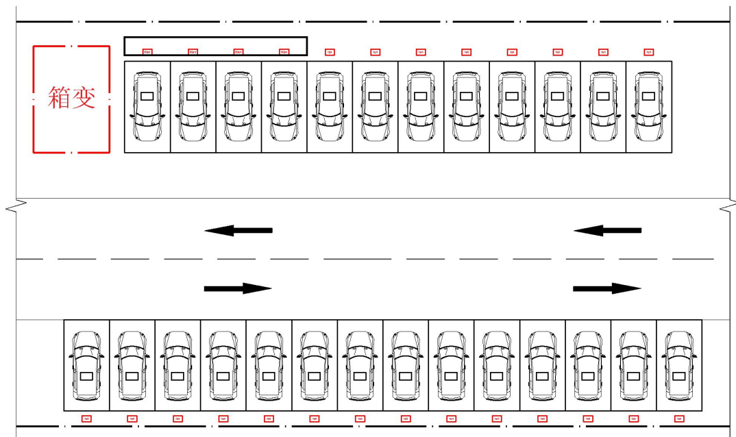
图 8 居民地上共享充电站布置图
