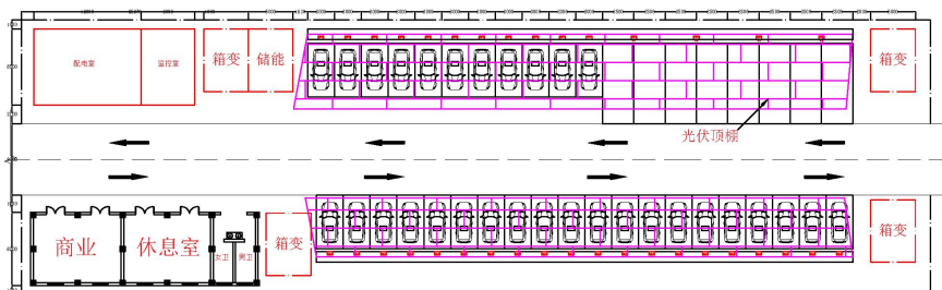
图 1 “光储充一体化”充电站 布置图
